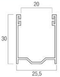
Guida in alluminio GUIDAL30x25
