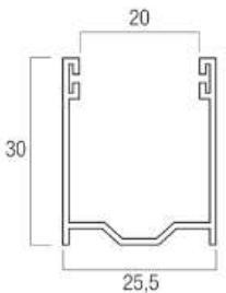
Guida in alluminio GUIAL30x25
