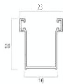
Guida in alluminio GUIAL28x16
