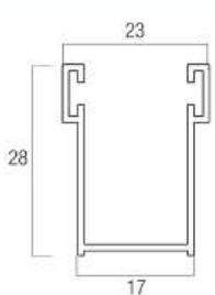
Guida in alluminio GUIAL28x17
