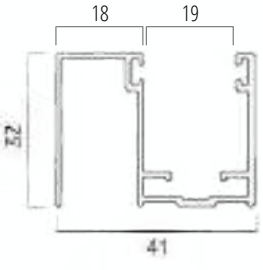
Guida in alluminio GUIDAL32x41 GUIDA DISTANZIALE
