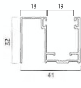
Guida in alluminio GUIAL32x41 DISTANZIALE
