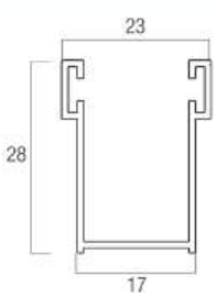
Guida in alluminio GUIDAL28x17
