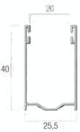
Guida in alluminio GUIDAL40x25
