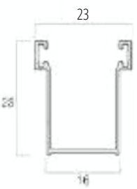
Guida in alluminio GUIDAL28x16
