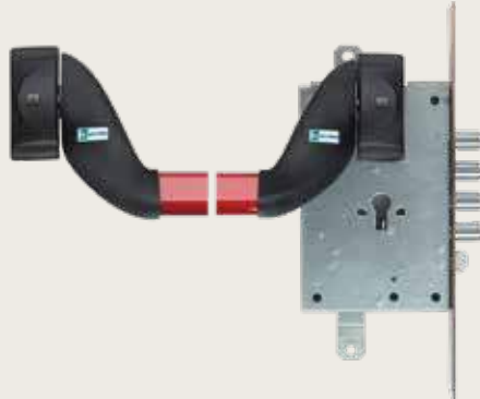
SERRATURA CON MANIGLIONE ANTI-PANICO LOCKING SYSTEM WITH PANIC EXIT DEVICE
